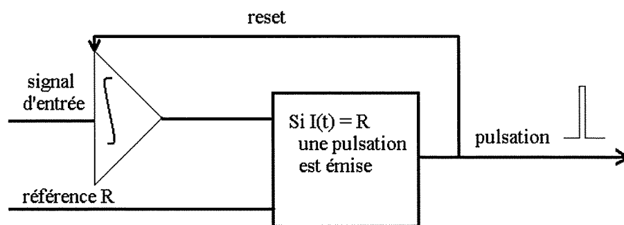
FIGURE 25 – Schéma de principe du générateur d'impulsions.
