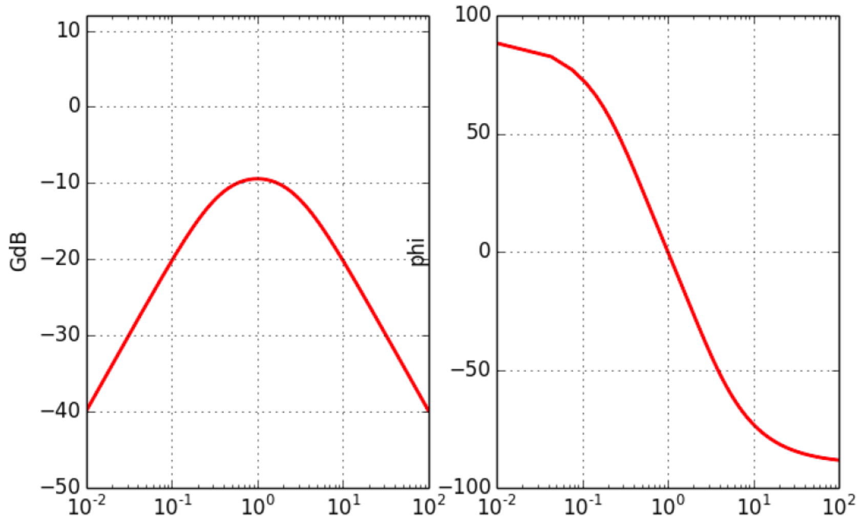
diagramme de Bode
