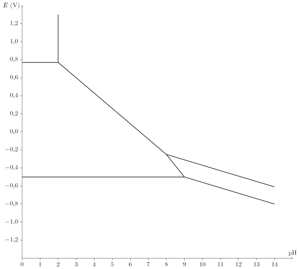
Figure B Diagramme potentiel-pH du fer
